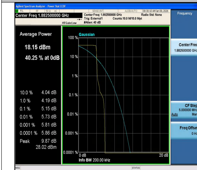
Band25-0.18-QPSK-26365-PASS
