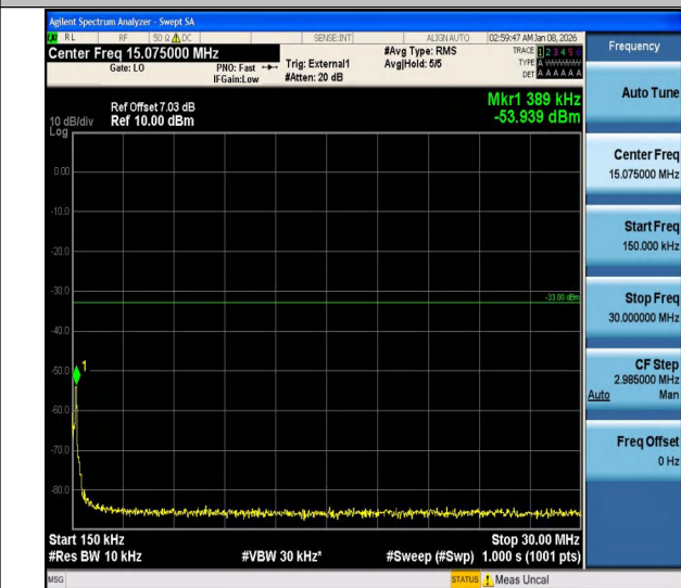
Band25-0.18-BPSK-26365-0.15-30-PASS
