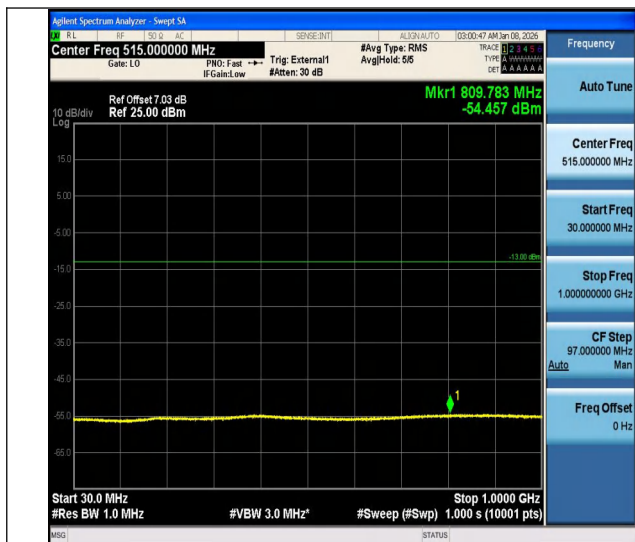
Band25-0.18-BPSK-26365-30-1000-PASS
