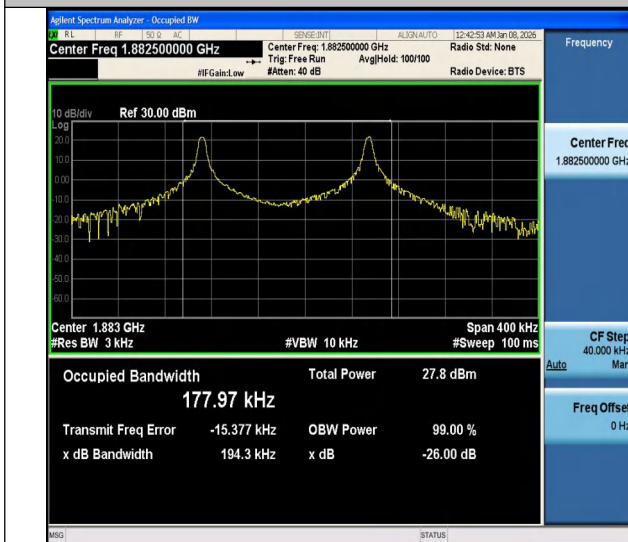
Band25-0.18-BPSK-26365-PASS
