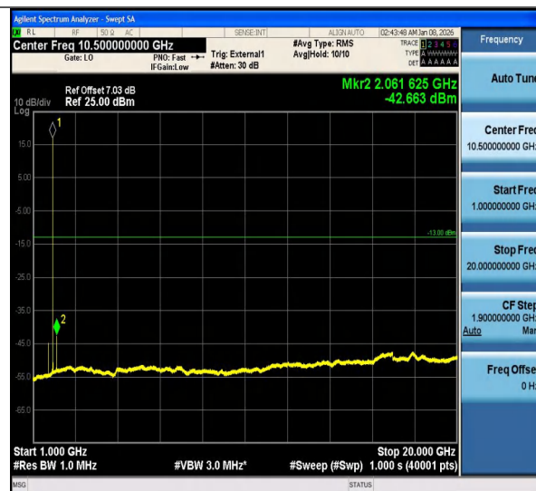
Band25-0.18-BPSK-26365-1000-20000-PASS
