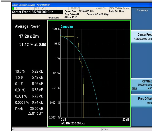
Band25-0.18-QPSK-26365-PASS
