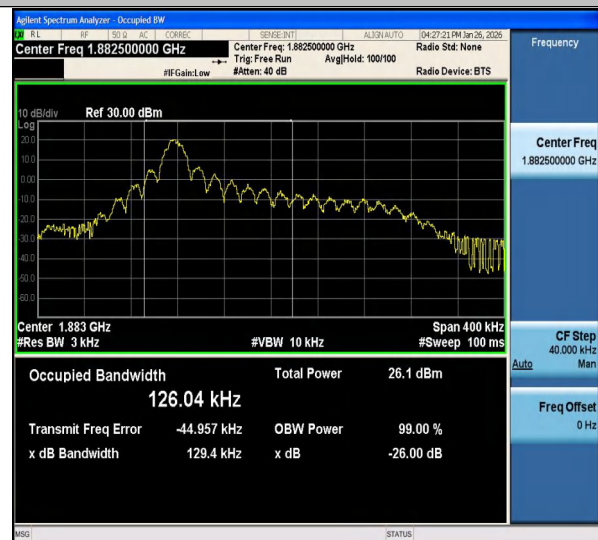
Band25-0.18-QPSK-26365-PASS
