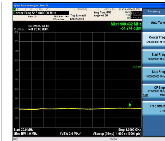
Band25-0.18-BPSK-26365-30-1000-PASS
