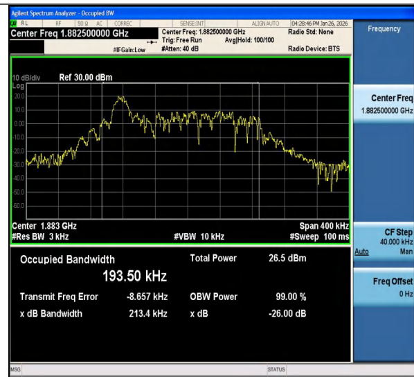
Band25-0.18-QPSK-26365-PASS
