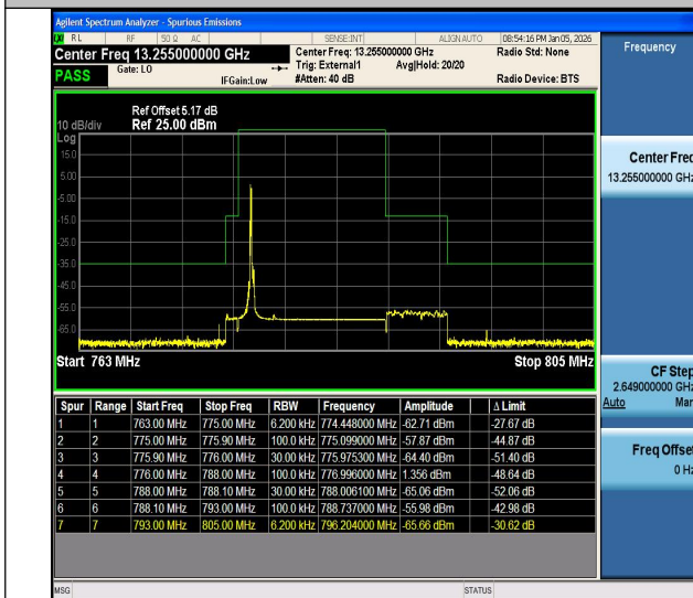
Band13-0.18-BPSK-23181-PASS
