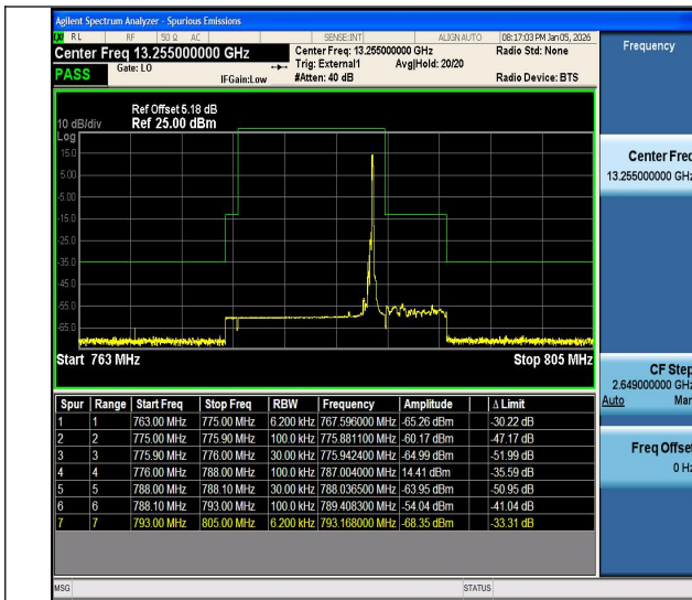
Band13-0.18-BPSK-23279-PASS
