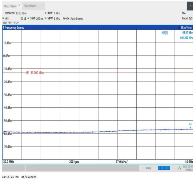
Band4-20MHz-QPSK-20050-PASS
