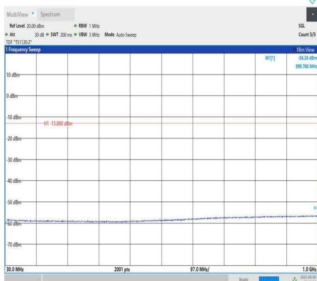
Band66-20MHz-QPSK-132072-PASS
