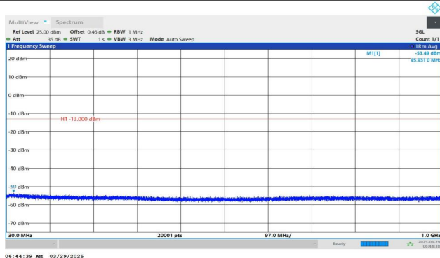
Band4-1312-2-30~1000MHz-PASS
