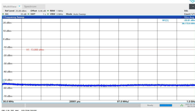
Band4-1413-5-30~1000MHz-PASS
