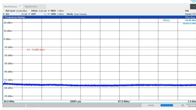
Band4-1413-3-30~1000MHz-PASS
