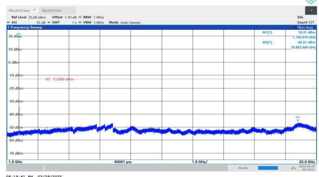
Band4-1413-5-1000~20000MHz-PASS
