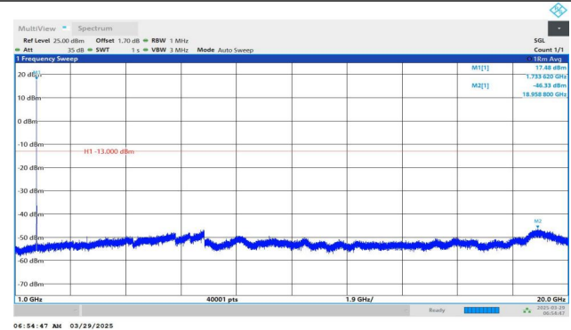
Band4-1413-4-1000~20000MHz-PASS
