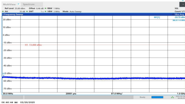
Band4-1312-3-30~1000MHz-PASS
