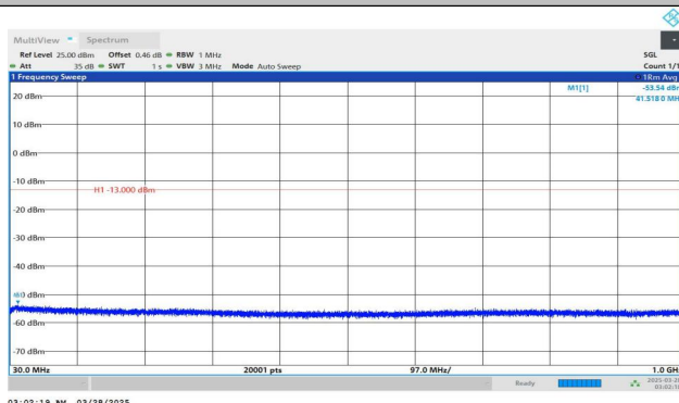
Band4-1413-30~1000MHz-PASS
