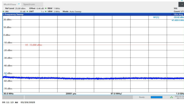
Band4-1413-2-30~1000MHz-PASS
