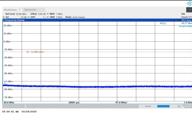
Band4-1413-4-30~1000MHz-PASS
