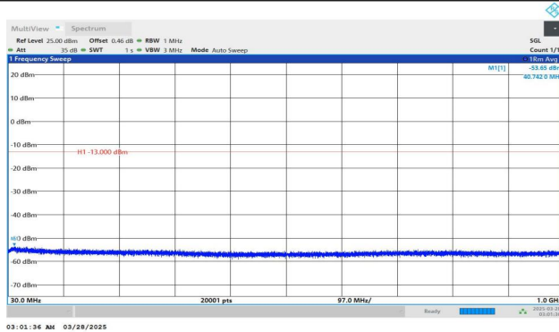
Band4-1312-30~1000MHz-PASS
