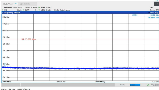
Band4-1513-2-30~1000MHz-PASS
