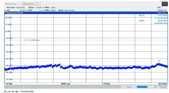
Band4-1312-5-1000~20000MHz-PASS
