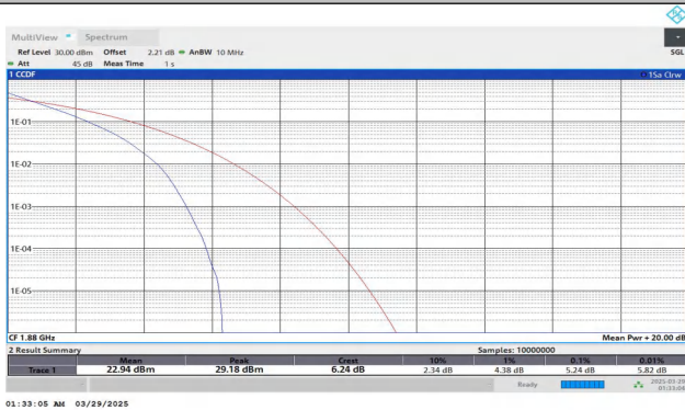
Band2-10MHz-QPSK-18900-50RB#0-PASS
