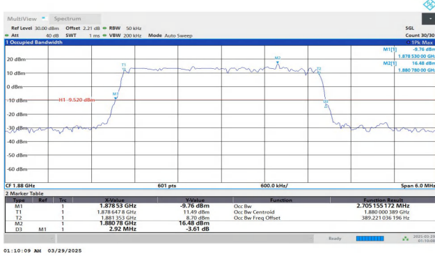
Band2-3MHz-QPSK-18900-15RB#0-PASS
