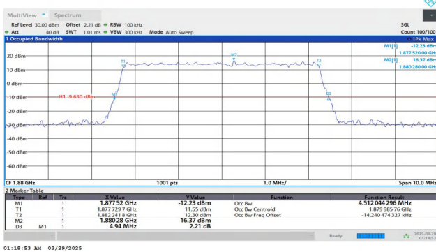
Band2-5MHz-QPSK-18900-25RB#0-PASS
