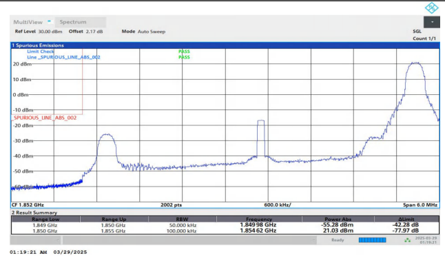
Band2-5MHz-QPSK-18625-1RB#24-PASS
