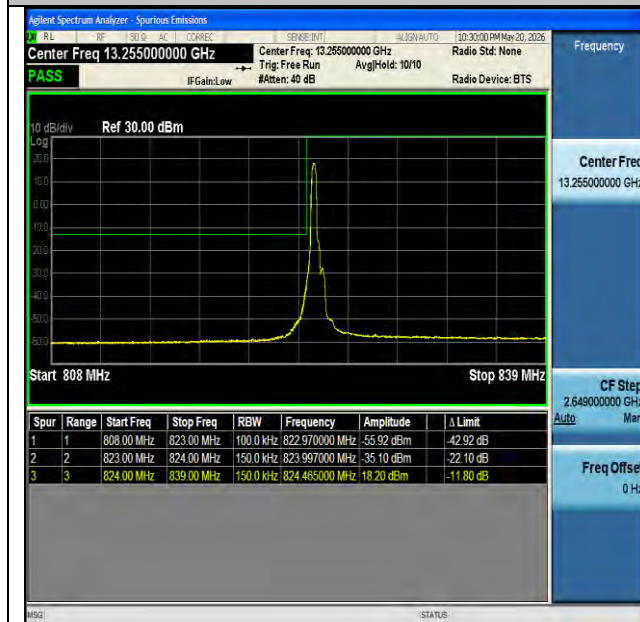
NTVN-n26(824-849)-PC3-15-15-L-CP-QPSK-Edge_1RB_Left-PASS
