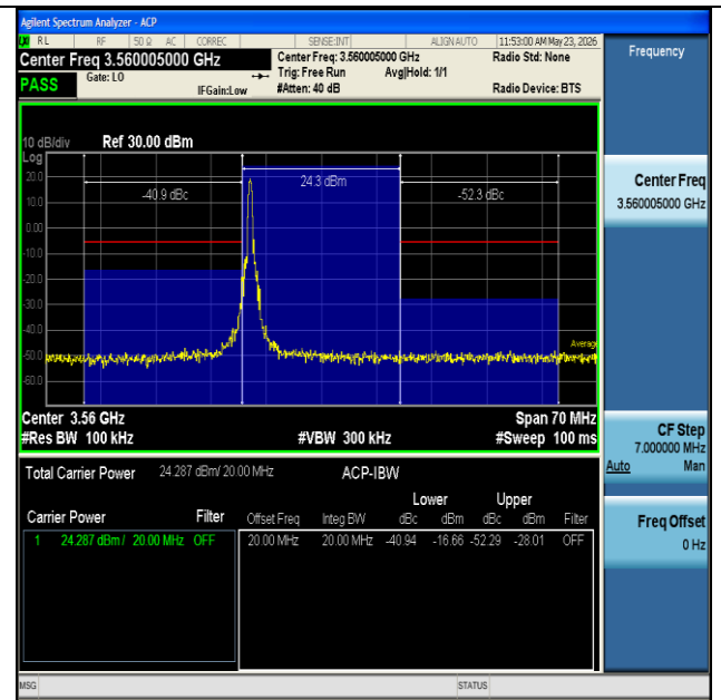
NTNV-n48-PC3-30-20-L-DFT-BPSK-Edge_1RB_Left-PASS
