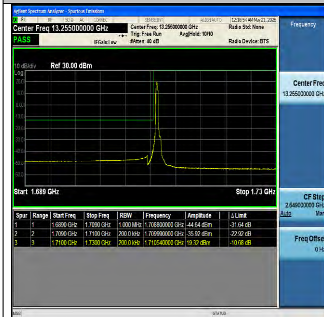
NTNV-n66-PC3-15-20-L-CP-QPSK-Edge_1RB_Left-PASS
