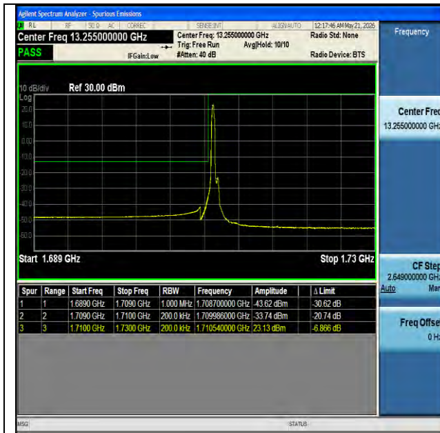
NTNV-n66-PC3-15-20-L-DFT-BPSK-Edge_1RB_Left-PASS
