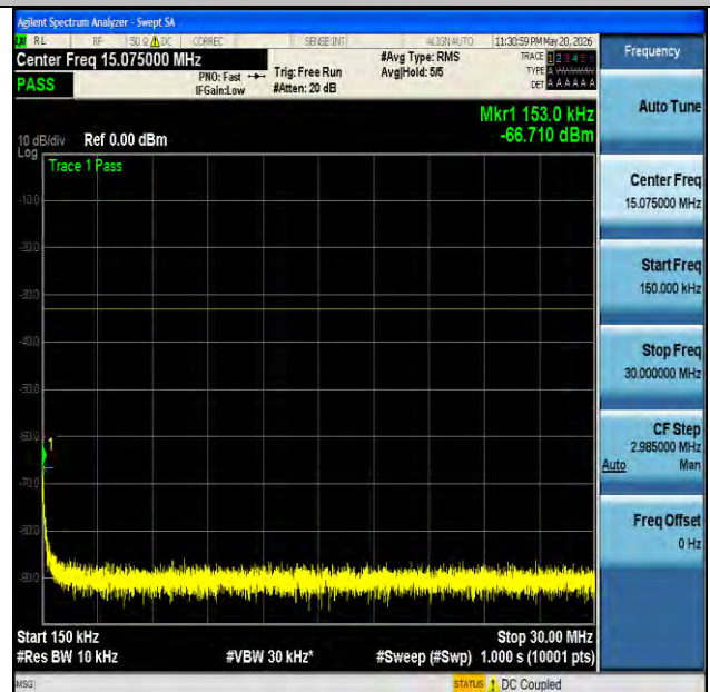
NTNV-n66-PC3-15-20-M-CP-QPSK-Edge_1RB_Left-0.15-30-PASS
