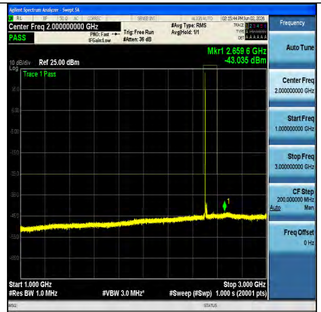
NTNV-n7-PC3-15-20-L-CP-QPSK-Edge_1RB_Left-1000-3000-PASS
