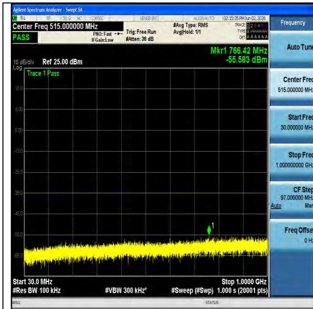
NTNV-n7-PC3-15-20-L-CP-QPSK-Edge_1RB_Left-30-1000-PASS
