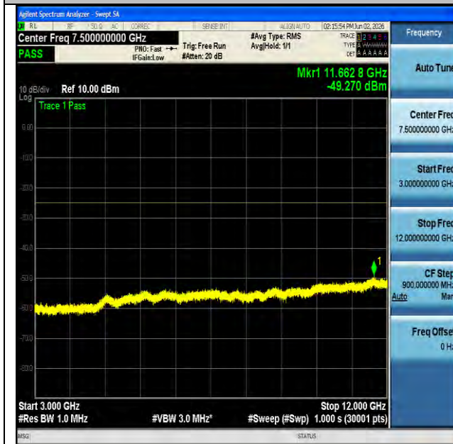
NTNV-n7-PC3-15-20-L-CP-QPSK-Edge_1RB_Left-3000-12000-PASS
