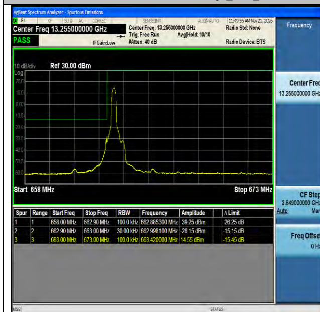
NTNV-n71-PC3-15-10-L-CP-QPSK-Edge_1RB_Left-PASS
