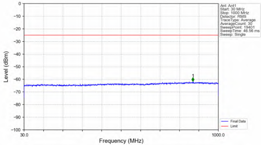
n7_15kHz_SISO_NTNV_20MHz_DFT-s-OFDM QPSK_2535MHz_Edge_1RB_Left_Ant1
