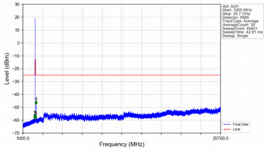
n7_15kHz_SISO_NTNV_20MHz_DFT-s-OFDM QPSK_2535MHz_Edge_1RB_Left_Ant1
