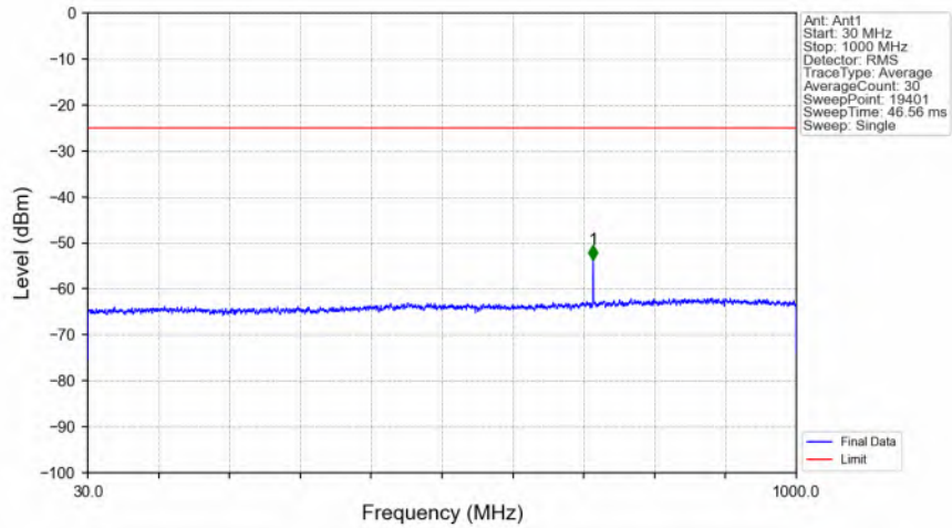
n7_15kHz_SISO_NTNV_5MHz_DFT-s-OFDM PI/2 BPSK_2535MHz_Edge_1RB_Left_Ant1
