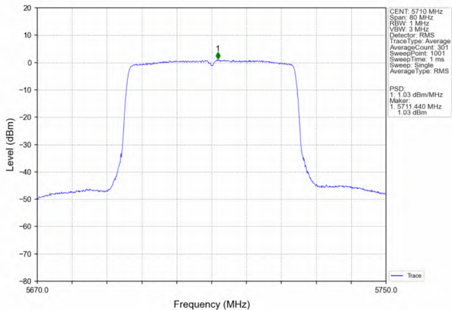
802.11ax(HEW40) HCH 5710MHz SU / Ant2 NTN
