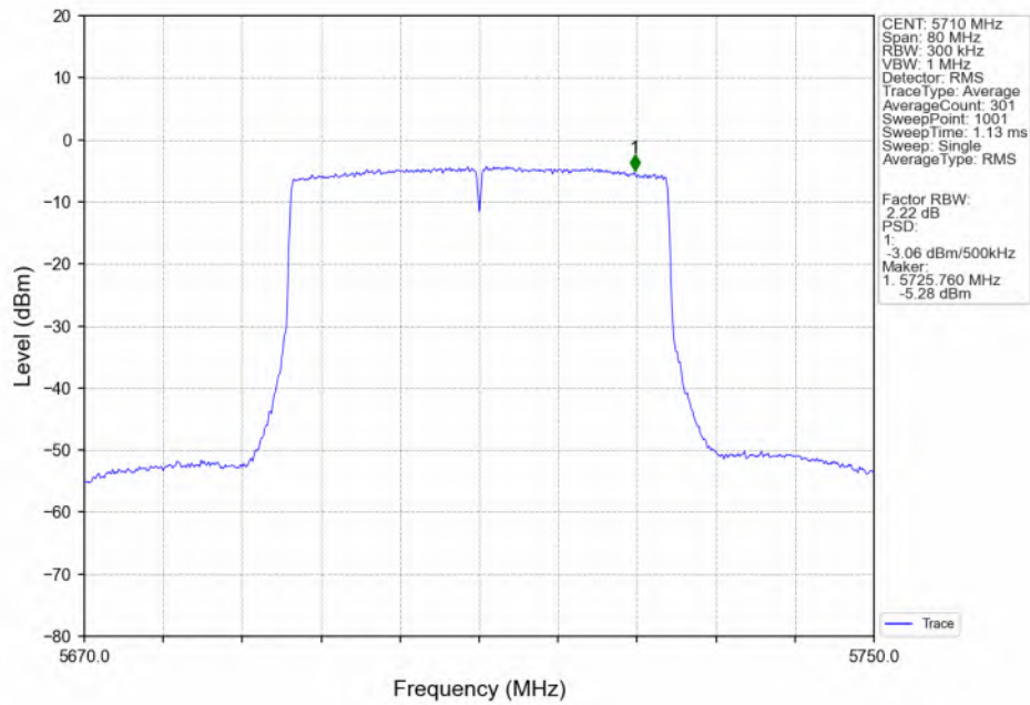
802.11ax(HEW40) HCH 5710MHz SU / MIMO NTN
