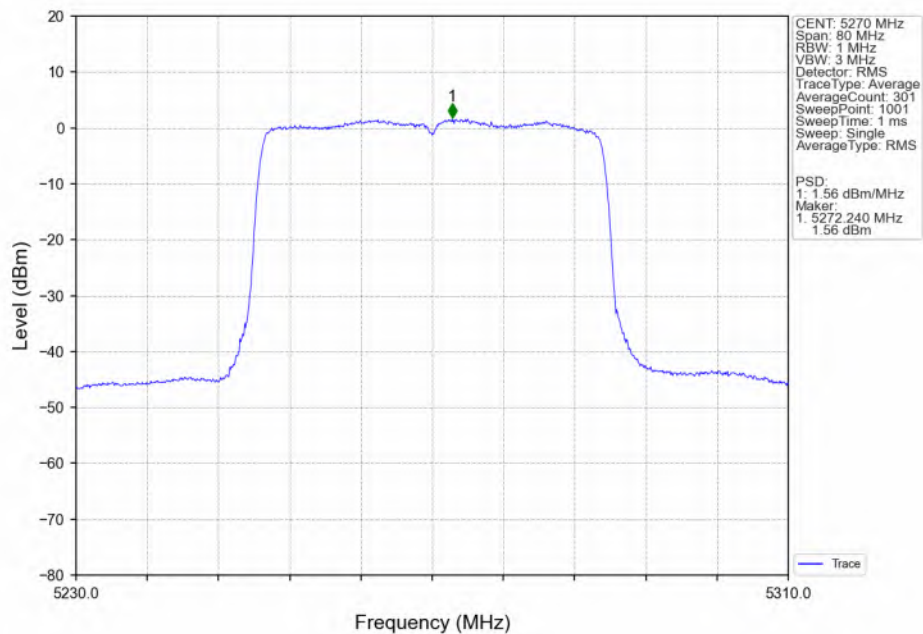
802.11ax(HEW40)_LCH_5270MHz_SU / Ant1_NTNV
