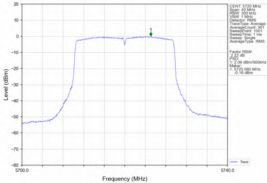
802.11ax(HEW20) HCH_5720MHz_SU / Ant2_NTNV
