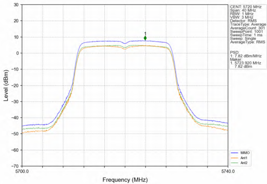
802.11n(HT20)_HCH_5720MHz_MIMO_NTNV
