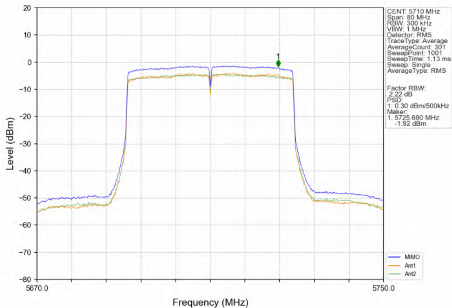
802.11ax(HEW40) HCH 5710MHz SU / MIMO NTN
