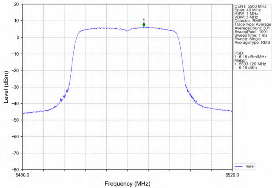
802.11ax(HEW20)_LCH_5500MHz_SU / Ant2_NTNV
