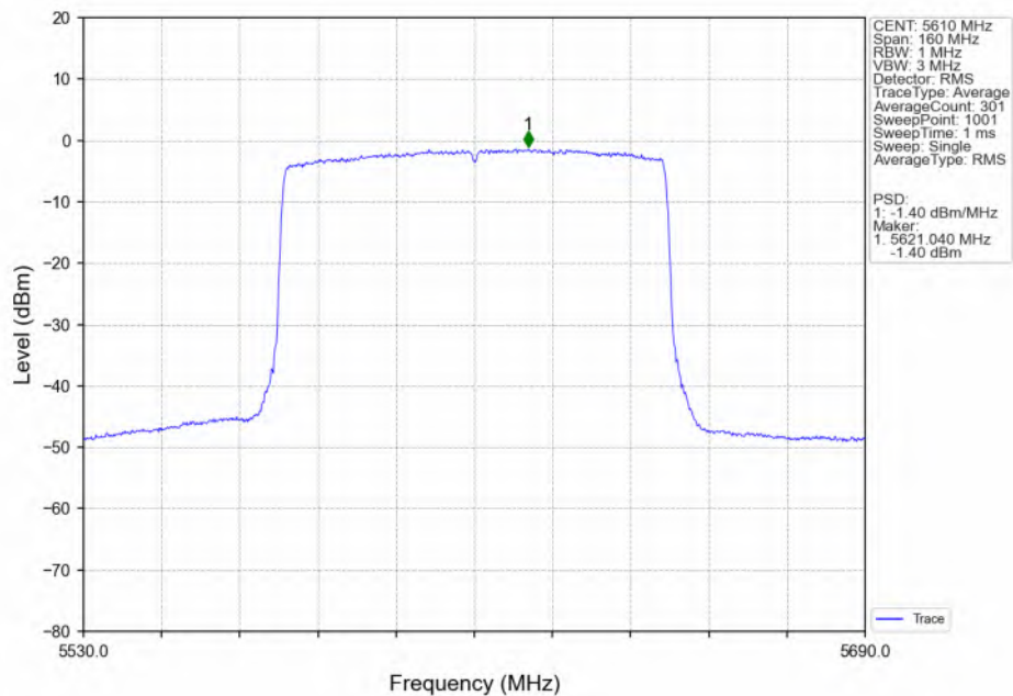
802.11ax(HEW80) HCH_5610MHz_SU / Ant2_NTNV
