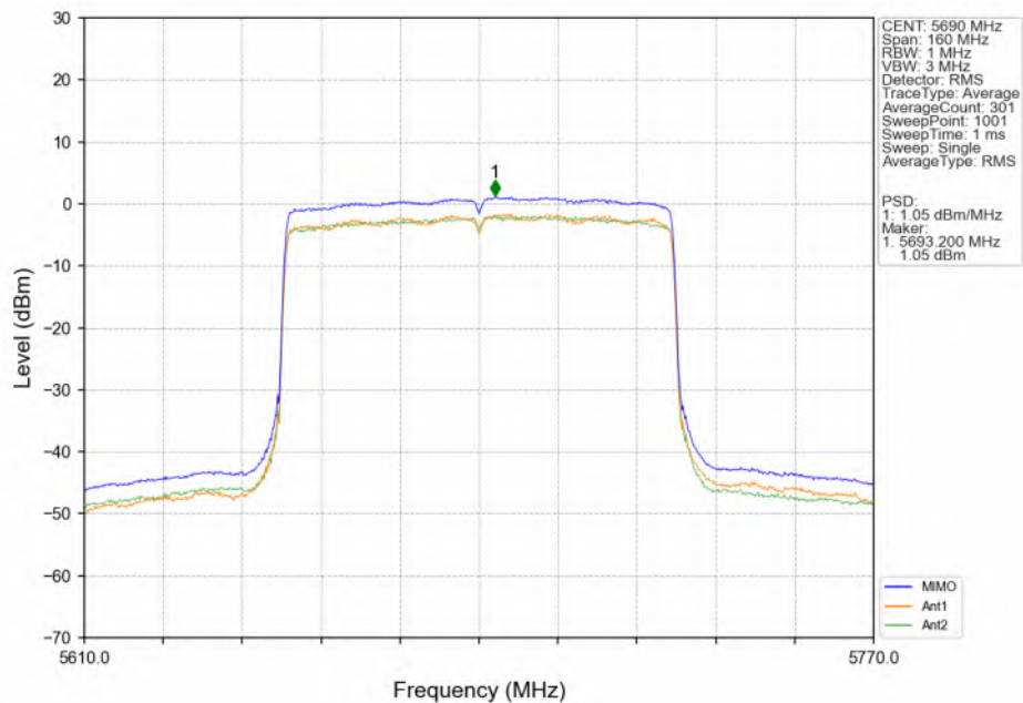
802.11ax(HEW80) HCH 5690MHz SU / MIMO NTN
