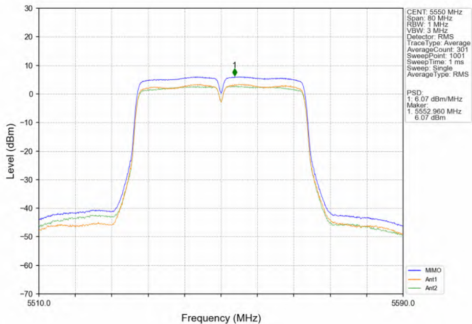
802.11n(HT40)_MCH_5550MHz_MIMO_NTNV
