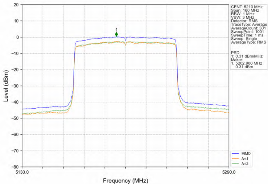
802.11ax(HEW80)_MCH_5210MHz_SU / MIMO_NTNV
