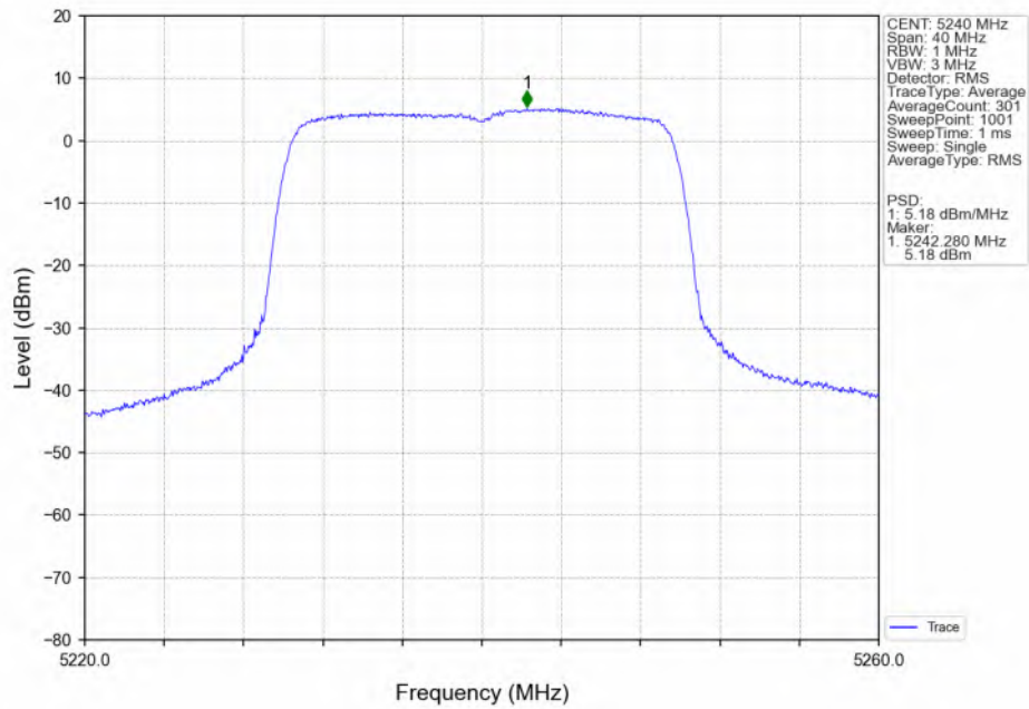
802.11ax(HEW20) HCH 5240MHz SU / Ant2 NTN
