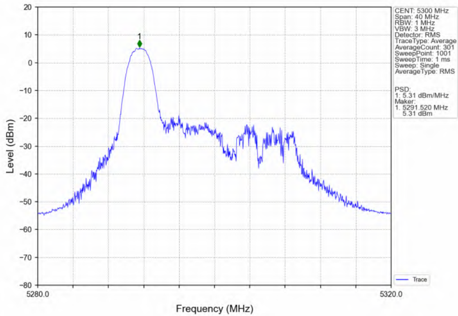
802.11ax(HEW20)_MCH_5300MHz_RU26_MIMO_NTNV
