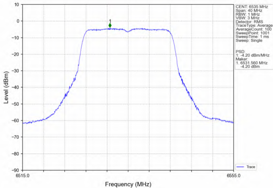
802.11a_LCH_6535MHz_Ant2_NTNV
