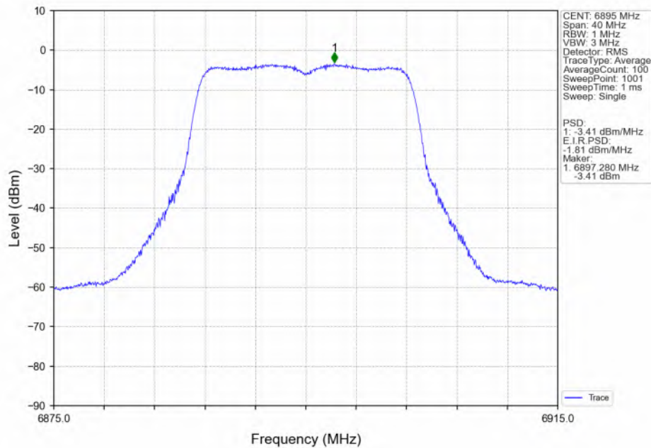
802.11a_LCH_6895MHz_Ant2_NTNV
