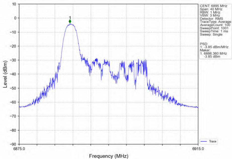
802.11ax(HEW20)_LCH_6895MHz_RU26_Ant1_NTNV
