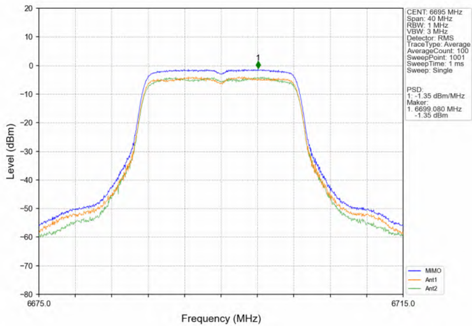
802.11a_MCH_6695MHz_MIMO_NTNV
