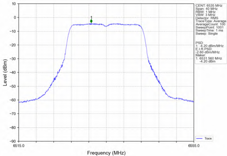
802.11a LCH 6535MHz Ant2 NTN
