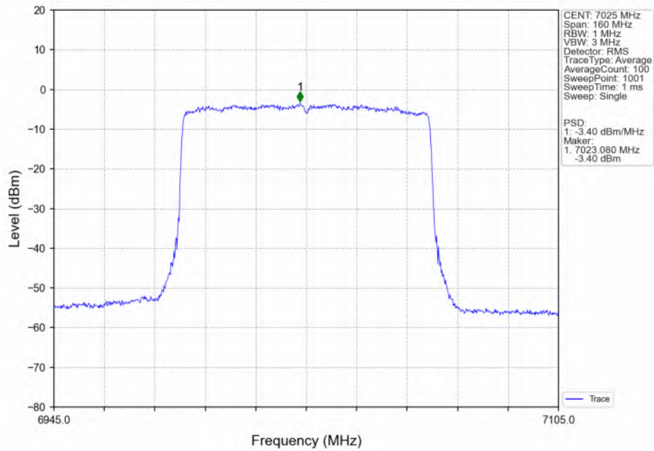
802.11ax(HEW80) HCH 7025MHz SU / MIMO NTN
