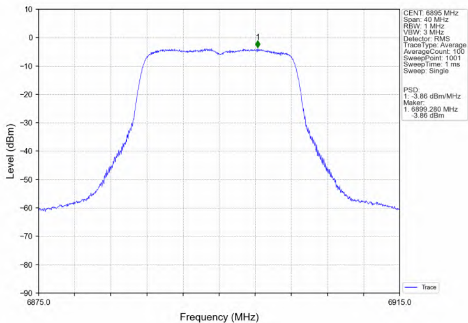
802.11a_LCH_6895MHz_Ant2_NTNV
