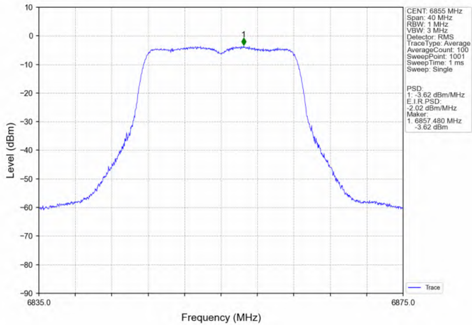
802.11a_HCH_6855MHz_Ant2_NTNV
