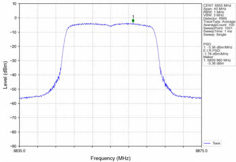
802.11ax(HEW20) HCH 6855MHz SU / Ant2 NTN
