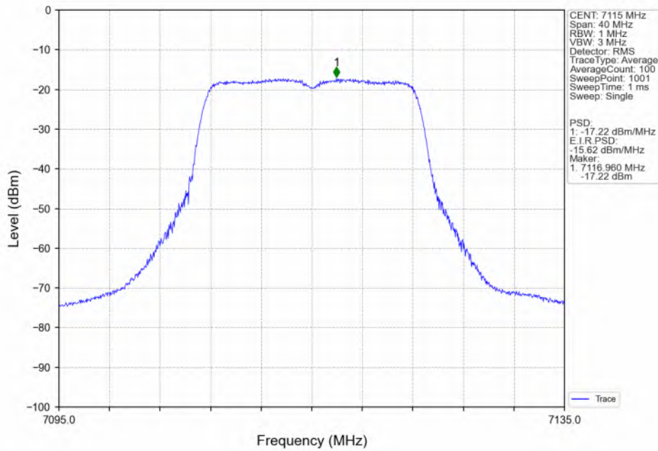
802.11a_HCH_7115MHz_Ant2_NTNV
