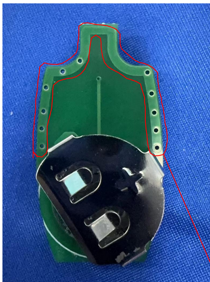
antenna
