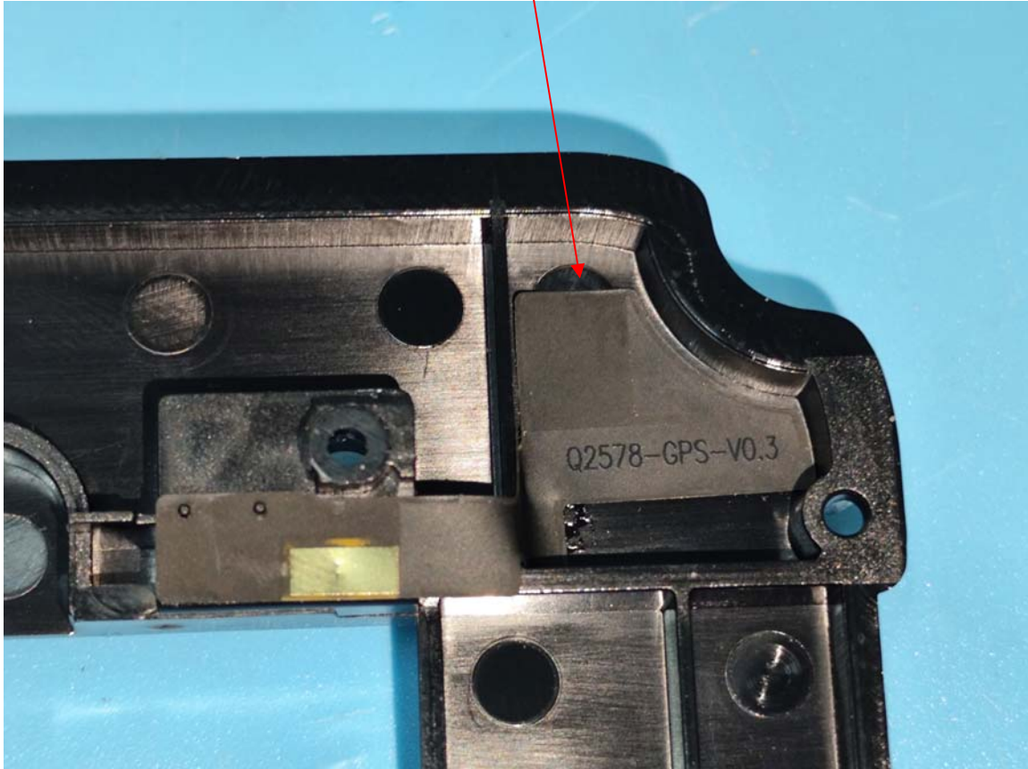
GPS Antenna
