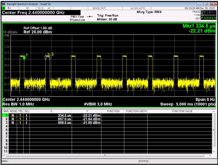
TX CH 19
