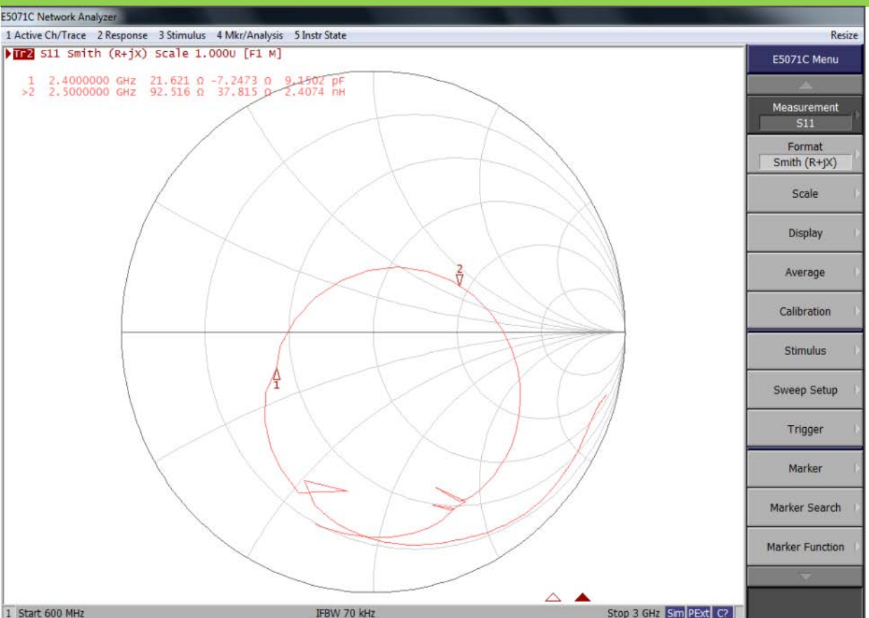
BT天线-S11
