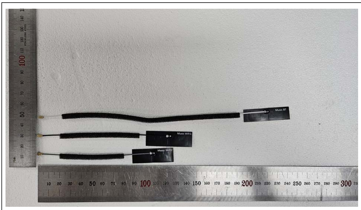
< M5 Antennas >
