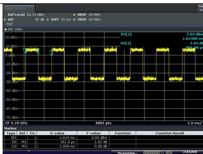
11ax_HE40
