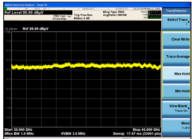
30 GHz ~ 40 GHz
