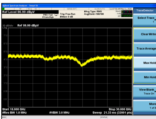
18 GHz ~ 30 GHz
