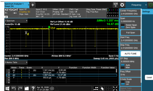
802.11n(HT20) (MCS0)
