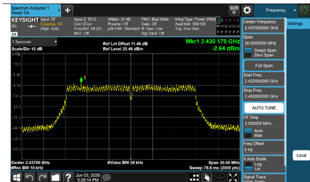
802.11n_HT20-CH 6
