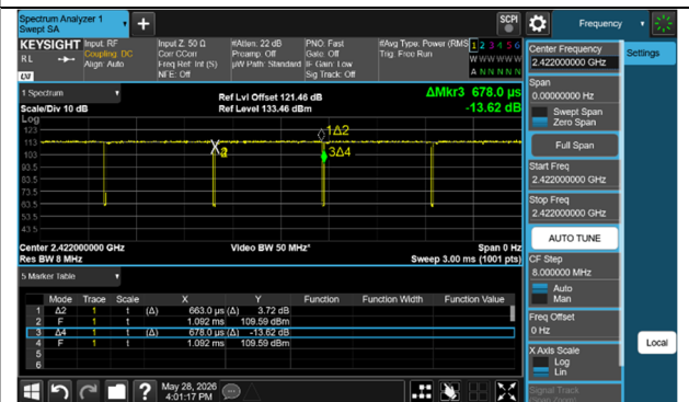
802.11n(HT40) (MCS0)
