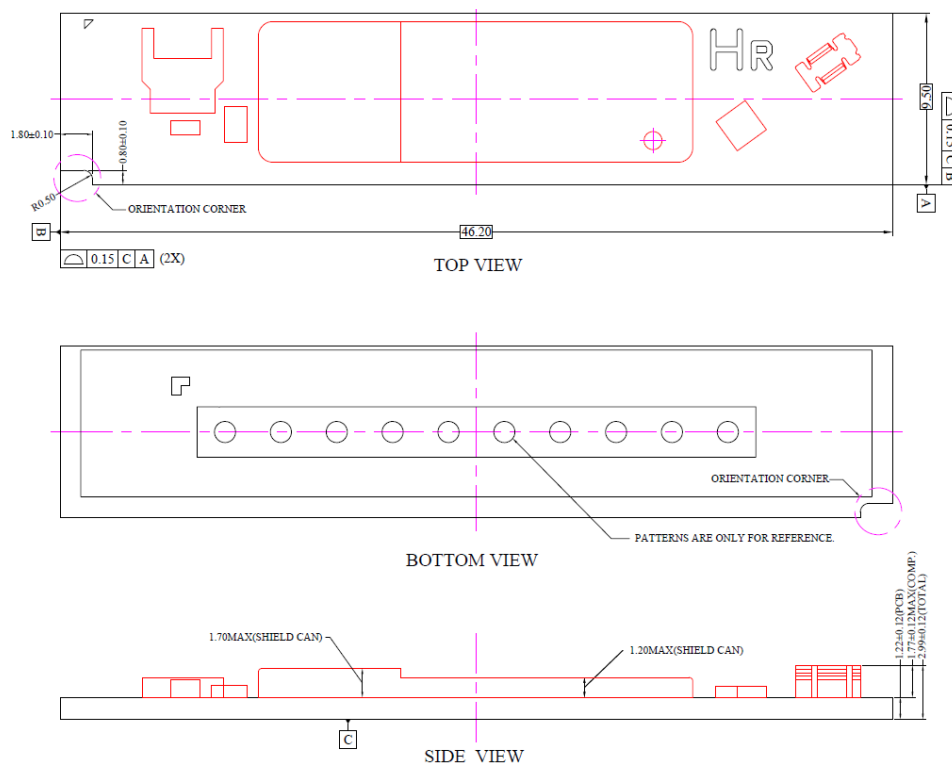
[Figure 5-4] 'LG2851 Slim-Right Display Module' Dimensions
