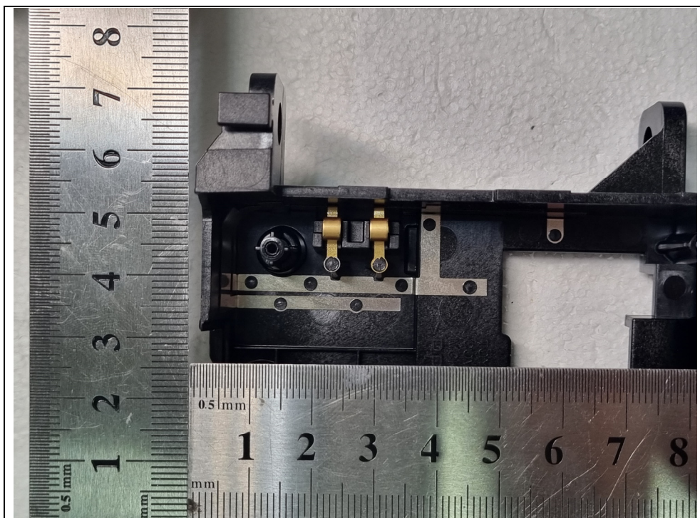
WWAN ANT 2
