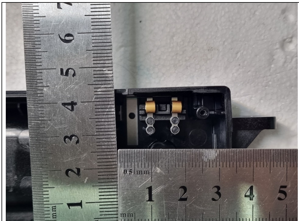
GNSS ANT
