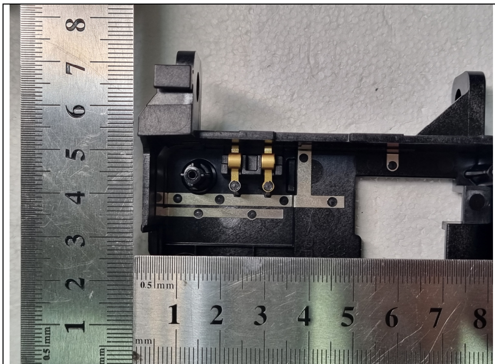
WWAN ANT 2
