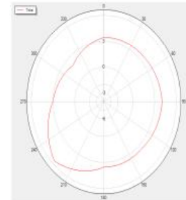
BLUETOOTH_Trp_V39 Total
