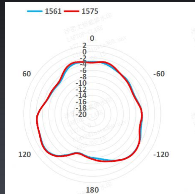
Phi=0° XOZ面
