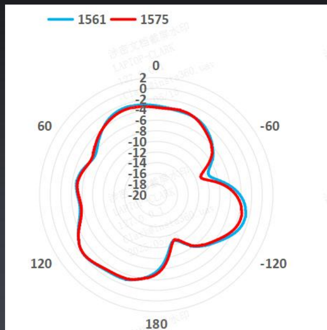
Phi=90° YOZ面
