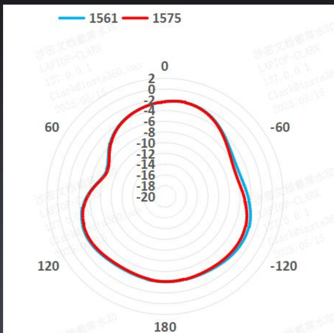
Theta=90° XOY面
