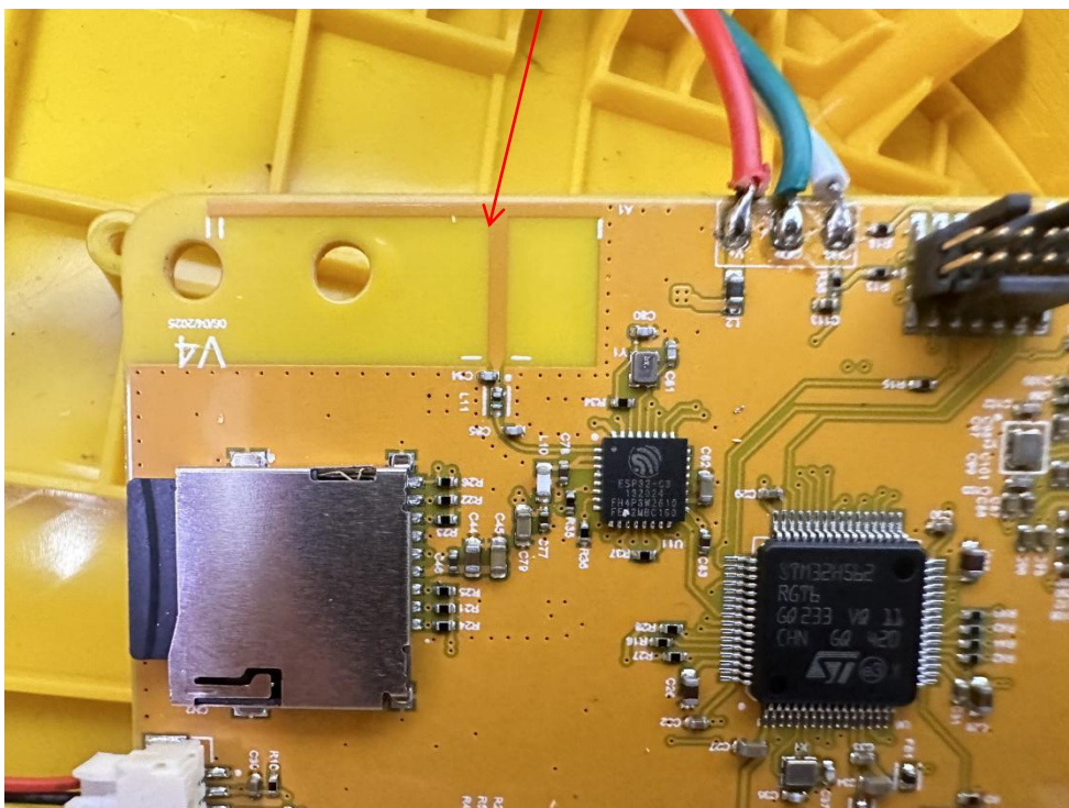
BT&WIFI ANT
