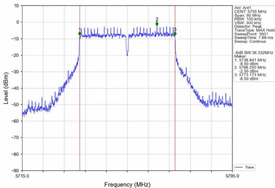
802.11ac(VHT40)_LCH_5755MHz_Ant1_NTNV
