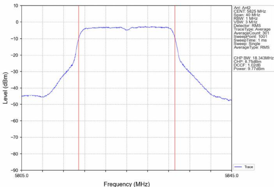
802.11n(HT20)_HCH_5825MHz_Ant2_NTNV
