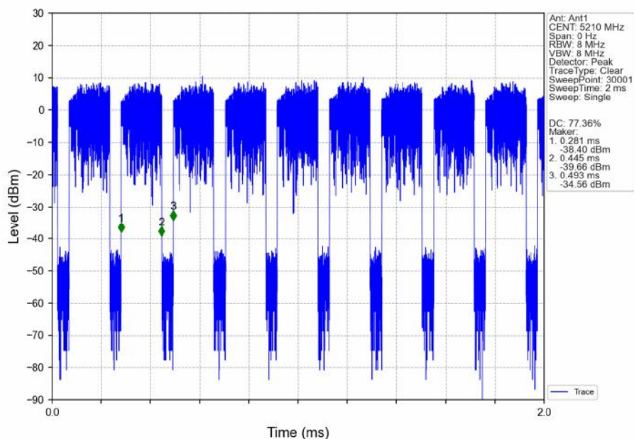
802.11ac(VHT80)_MCH_5210MHz_Ant1_NTNV
