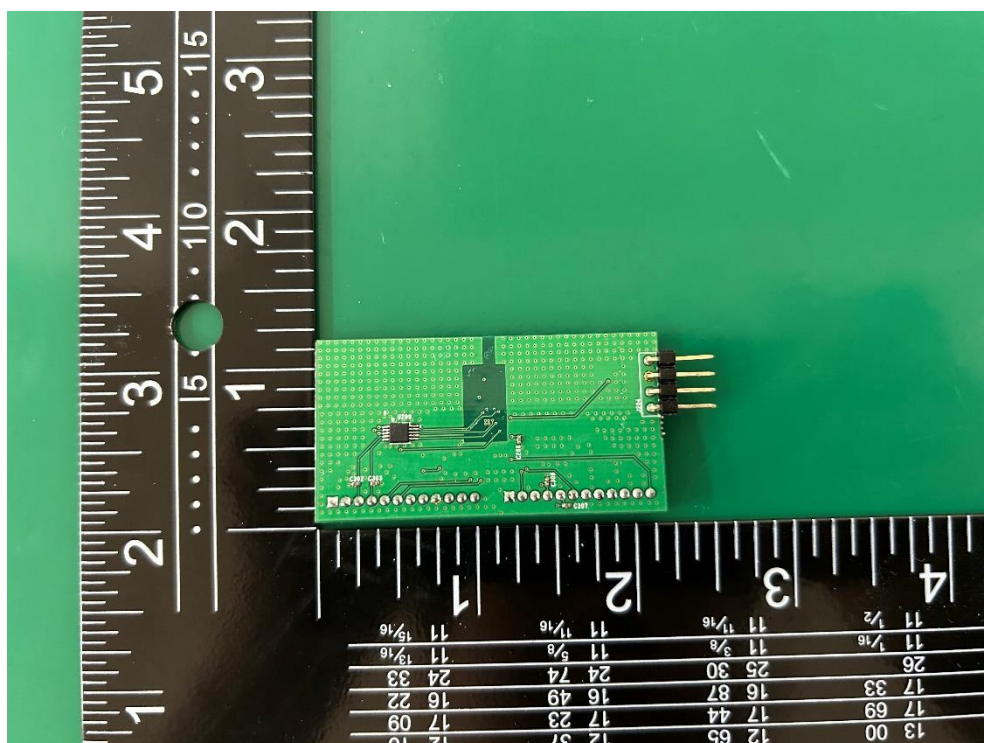
BLE Board Bottom
