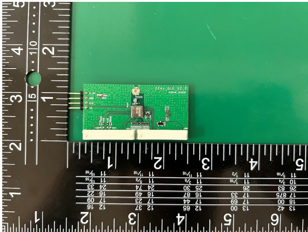
BLE Board Top
