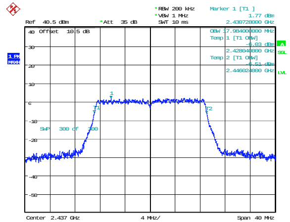
802.11n20_2437MHz
