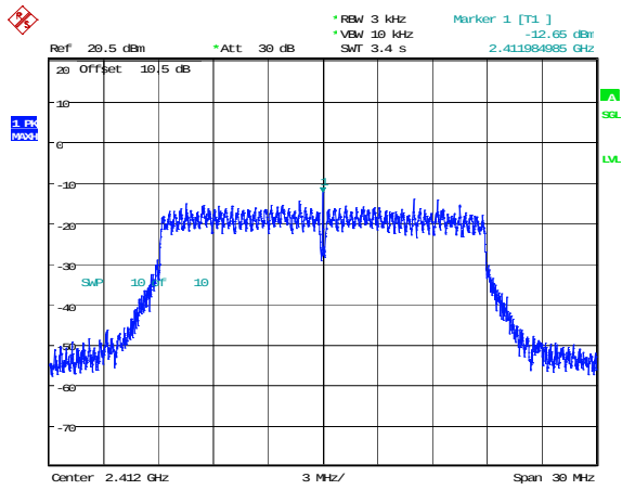
802.11n20_2412MHz
