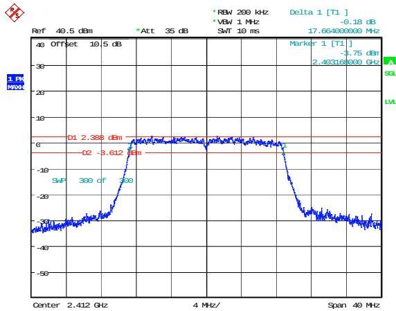
802.11n20_2412MHz
