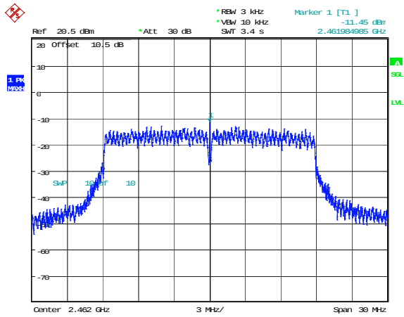
802.11n20_2462MHz
