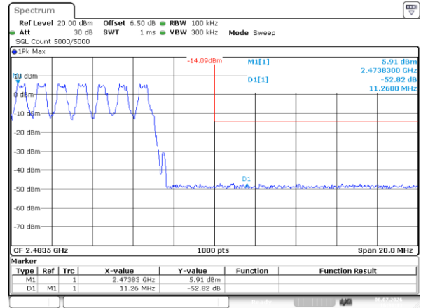
DH1_Hopping_Upper
