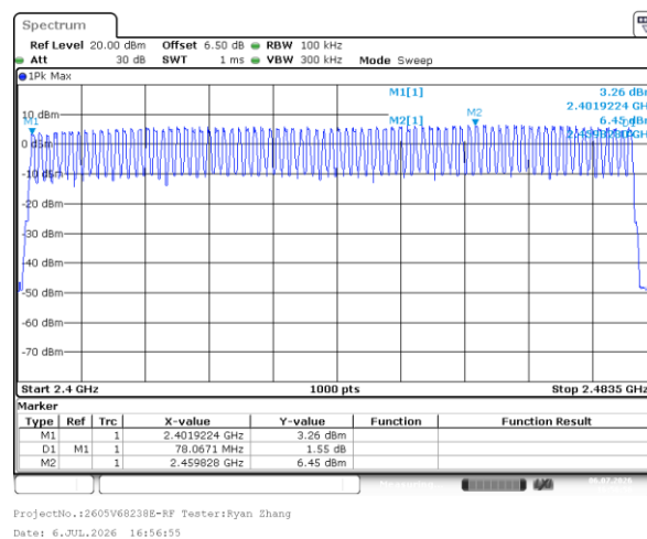
DH1_Hopping
