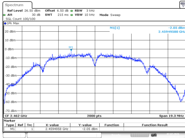
802.11b_2462MHz
