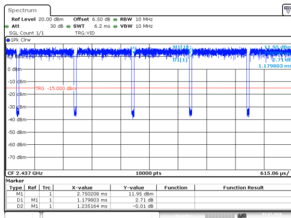
802.11n20_2437MHz
