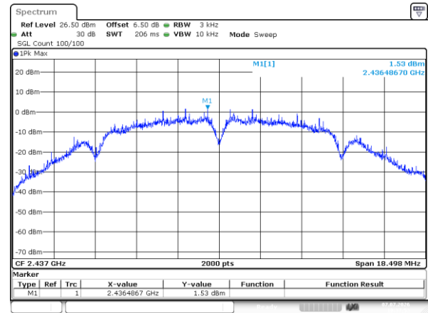
802.11b_2437MHz
