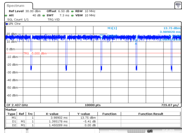
802.11g_2437MHz
