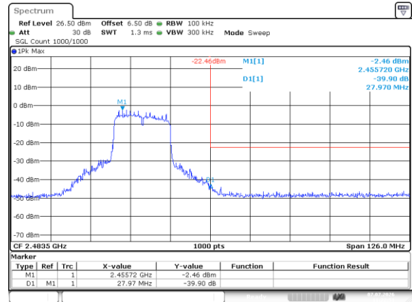
802.11n20_2462MHz
