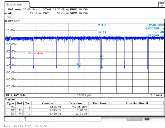
IEEE 802.11g_20MHz_Channel 11
