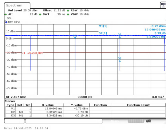
IEEE 802.11b_20MHz_Channel 6
