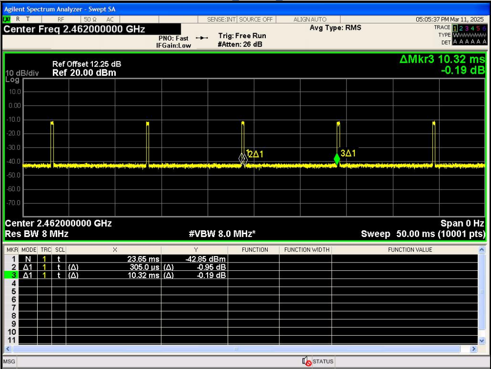
IEEE 802.11ax_20MHz_Channel 11
