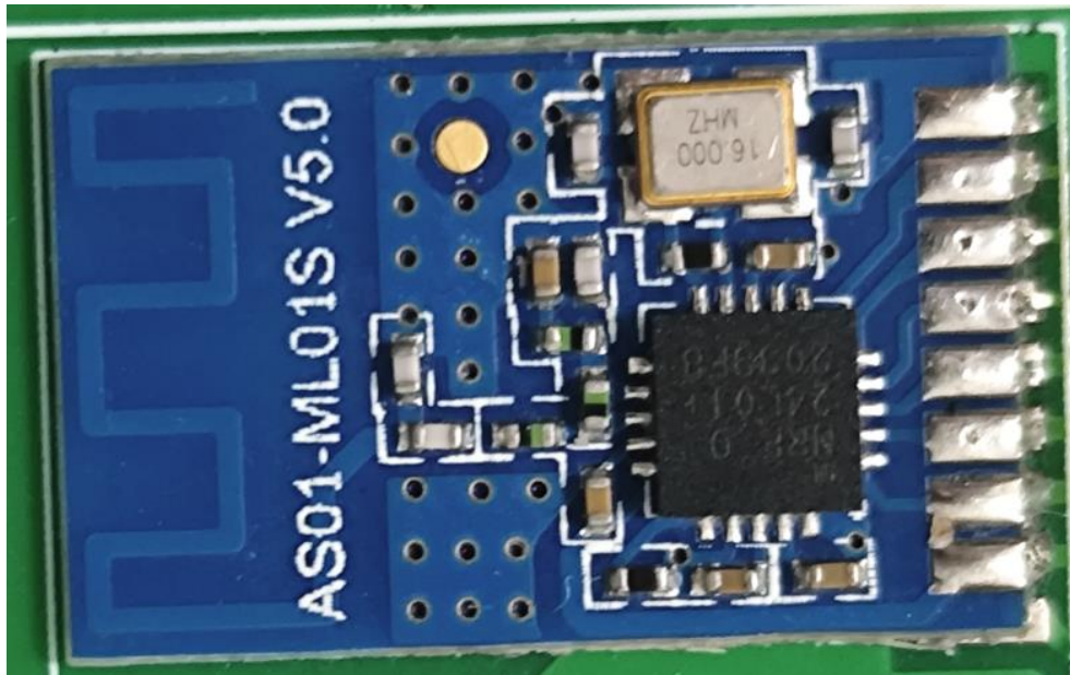
RF 2.4GHz module: AS01-ML01S
