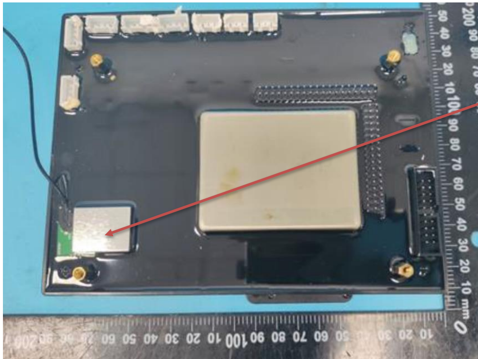
WIFI module: WT85R
