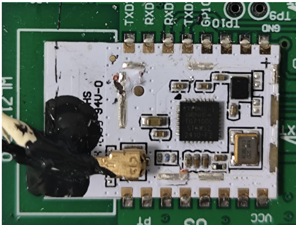
BLE module: WL71
