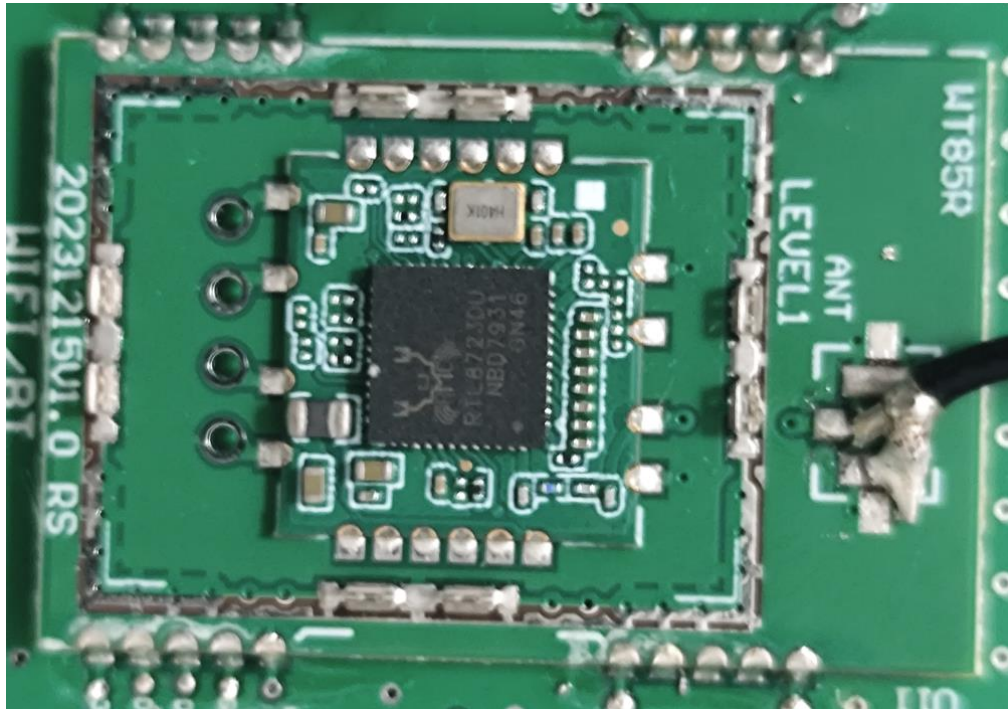
WIFI module: WT85R
