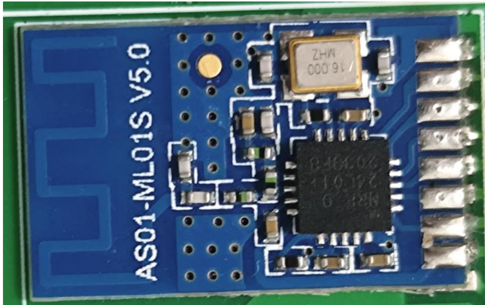
2.4GHz RF module: AS01-ML01S
