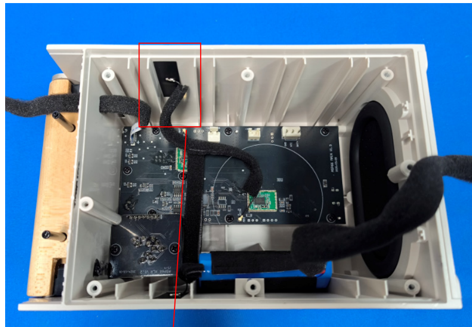
BDR/EDR/BLE Ant.
