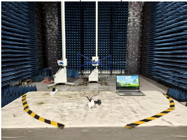
RE (Below 1GHz)
