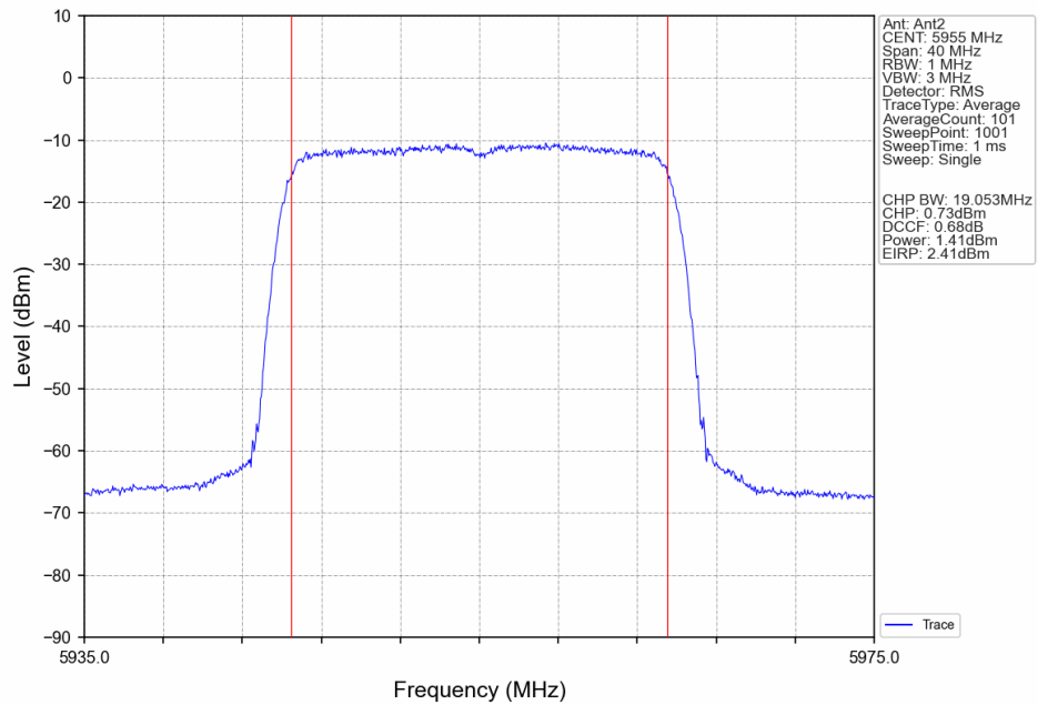
802.11be(EHT20)_LCH_5955MHz_SU_ / Ant2_NTNV
