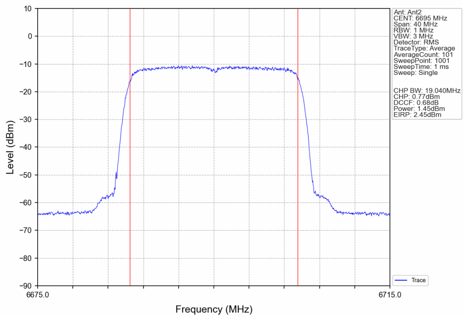
802.11be(EHT20) MCH 6695MHz SU / Ant2 NTN
