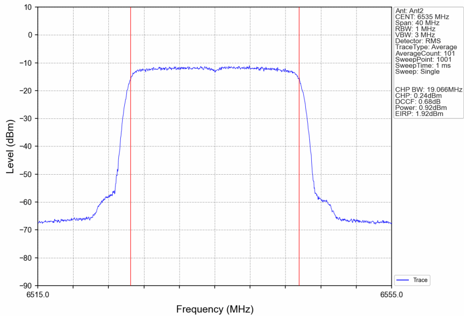
802.11be(EHT20) LCH 6535MHz SU / Ant2 NTN
