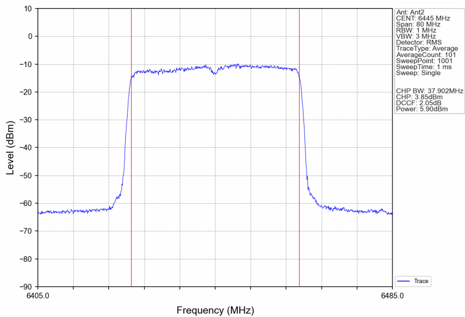
802.11be(EHT40) LCH 6445MHz SU / Ant2 NTN
