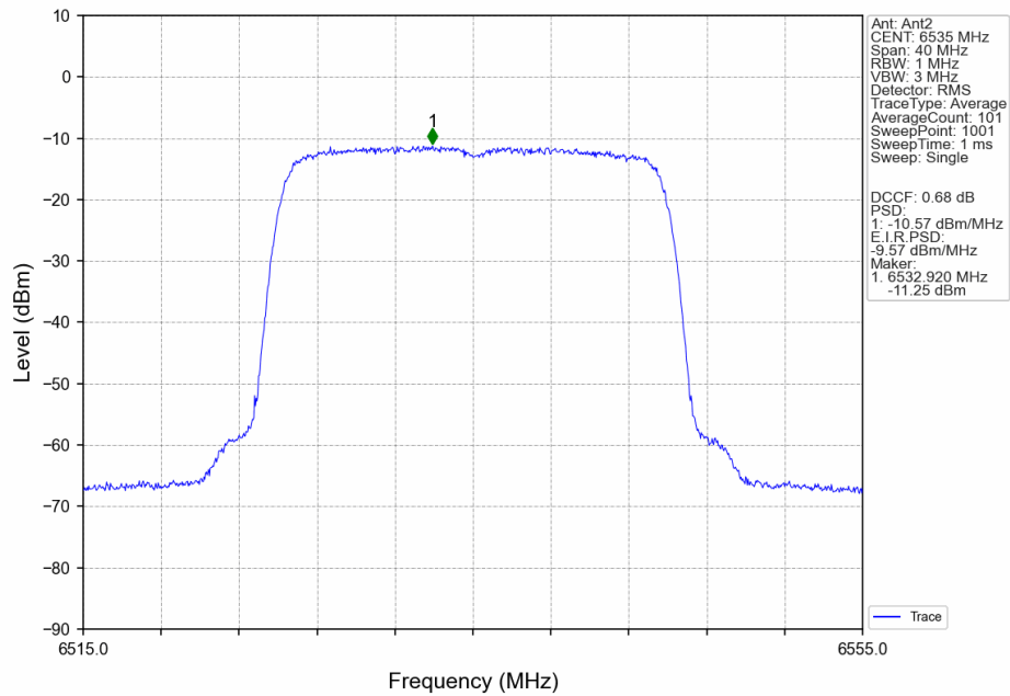
802.11be(EHT20) LCH 6535MHz SU / Ant2 NTN
