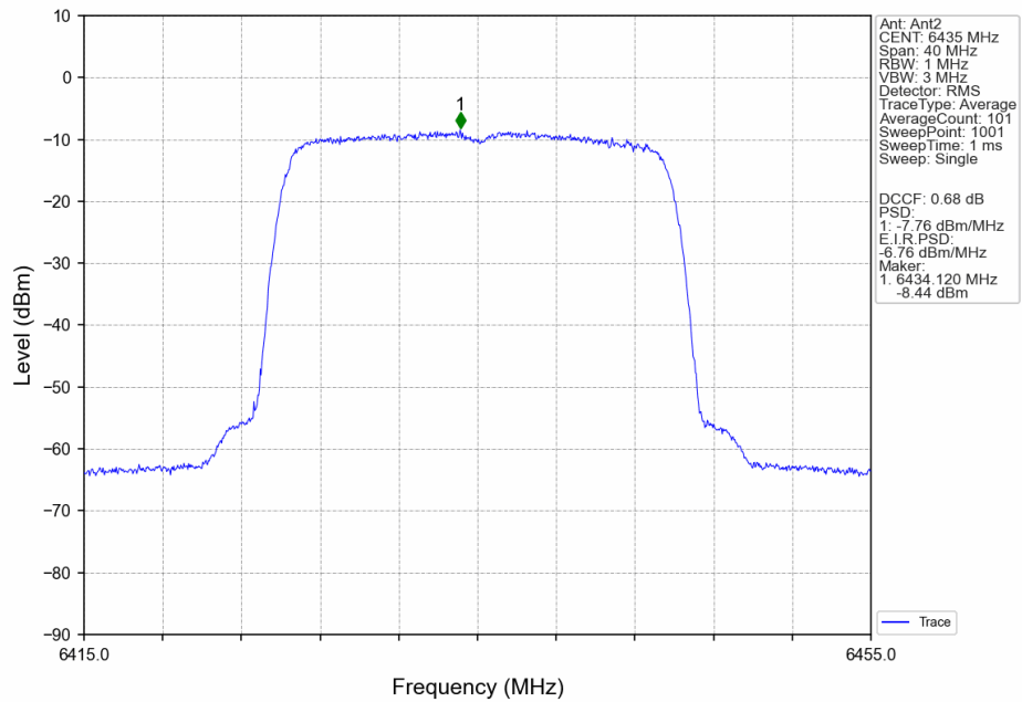
802.11be(EHT20) LCH 6435MHz SU / Ant2 NTN
