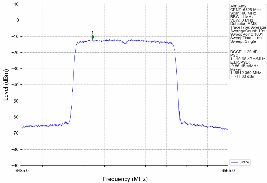
802.11be(EHT40) HCH 6525MHz SU / Ant2 NTN
