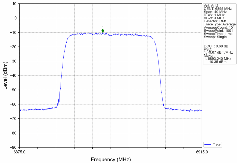
802.11be(EHT20) LCH 6895MHz SU / Ant2 NTN
