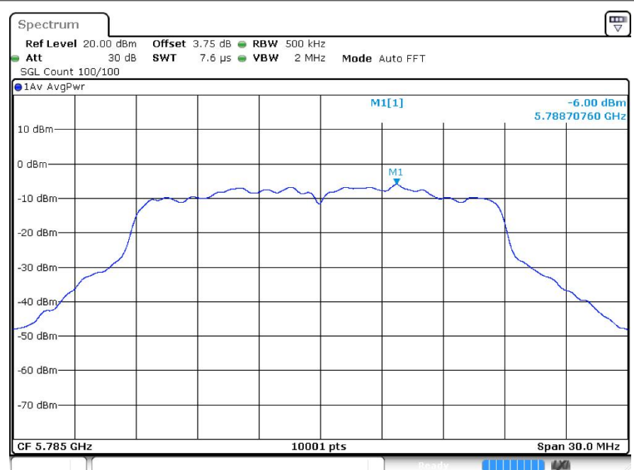
PSD ac20 5785MHz Ant1
