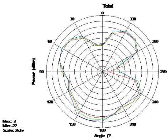
天线辐射方向图 Antenna Radiation Pattern
