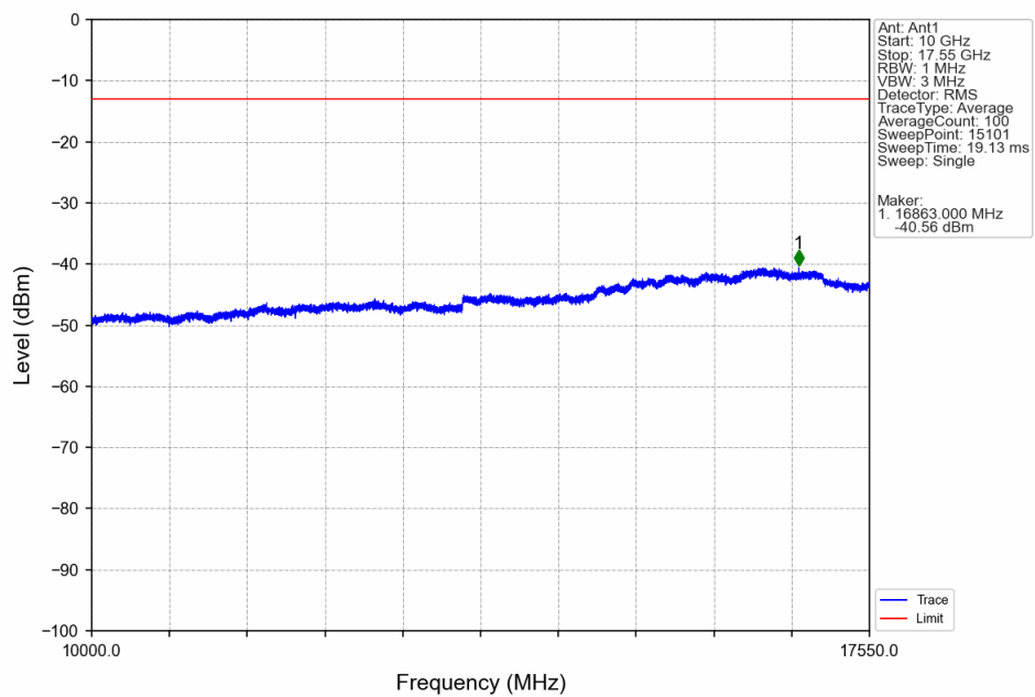
Band4_10MHz_QPSK_HCH_1750MHz_RB_1_0_NTNV
