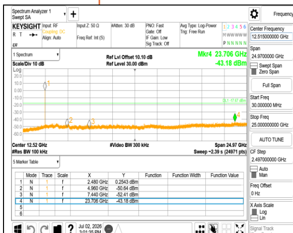
Spurious Emission BLE 1M 2480MHz
