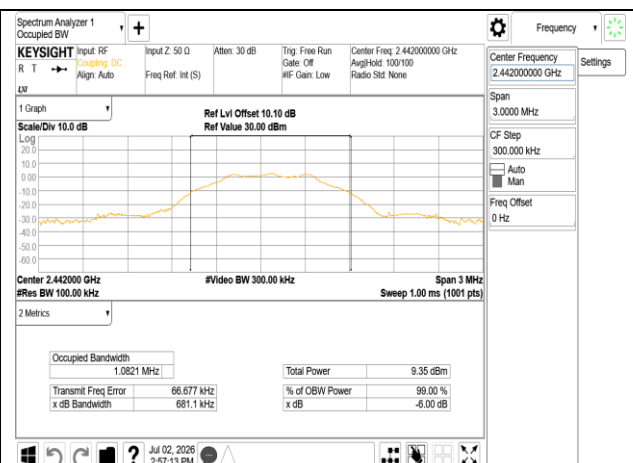
OBW 6dB BLE 1M 2442MHz
