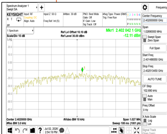
PSD BLE 1M 2402MHz
