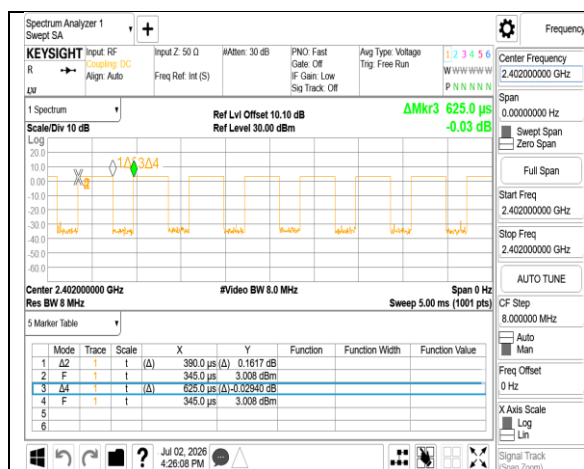
BLE_1M_2402MHz
