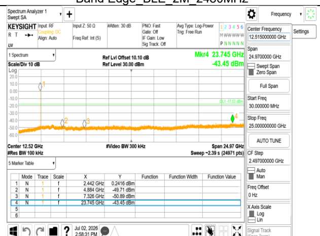
Spurious Emission BLE 1M 2442MHz
