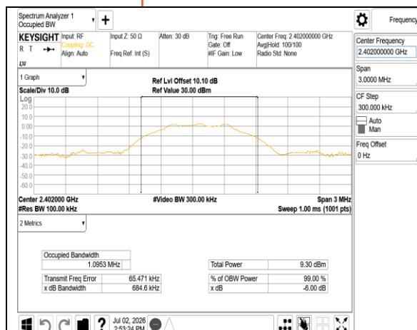
OBW 6dB BLE 1M 2402MHz
