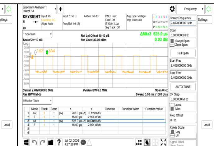
BLE_2M_2402MHz
