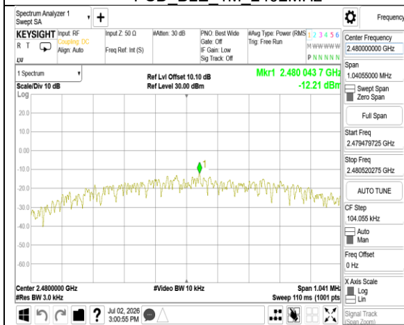
PSD BLE 1M 2480MHz
