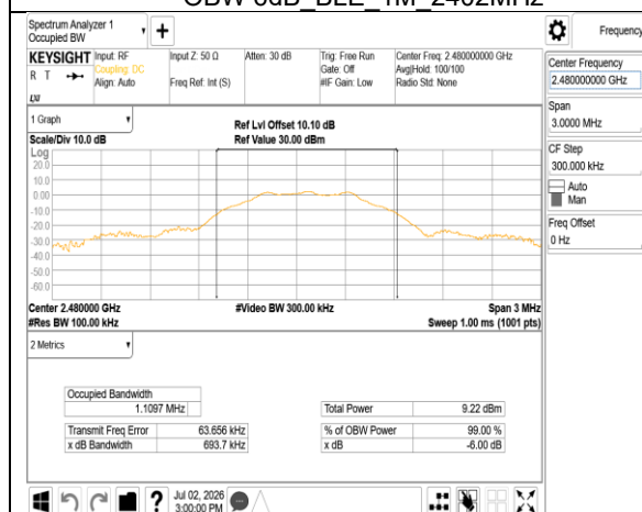
OBW 6dB BLE 1M 2480MHz
