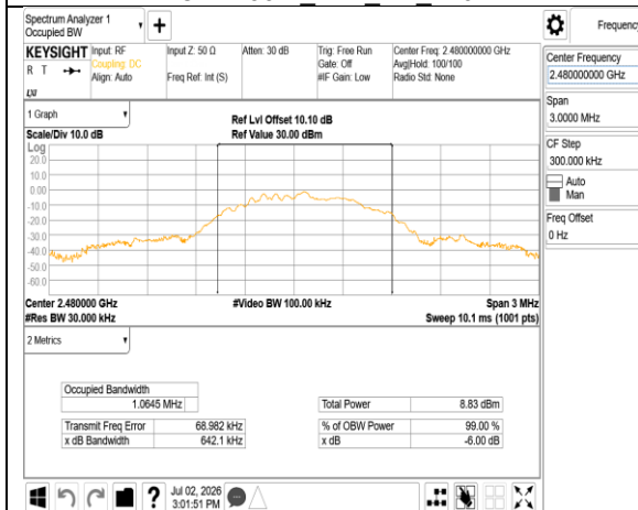
OBW 99% BLE 1M 2480MHz
