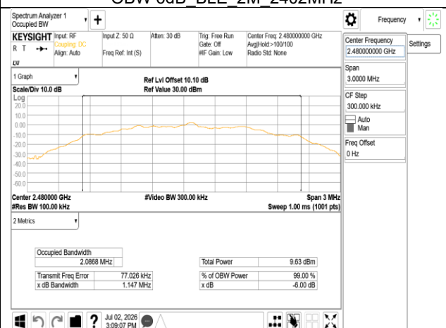
OBW 6dB BLE 2M 2480MHz
