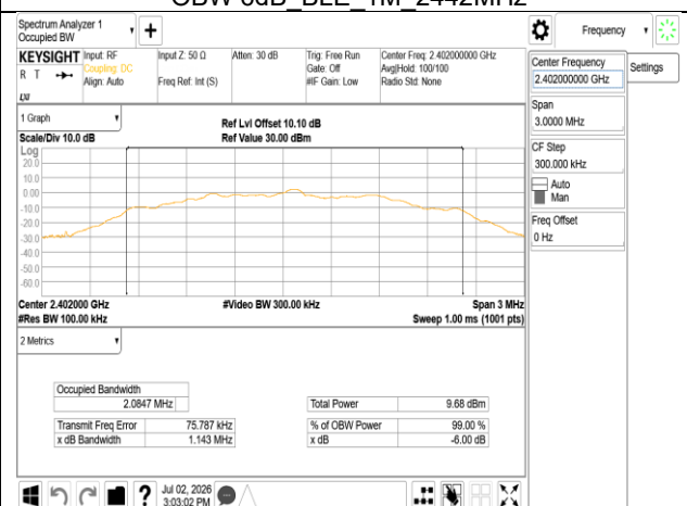
OBW 6dB BLE 2M 2402MHz
