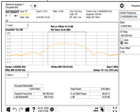
OBW 99% BLE 1M 2402MHz
