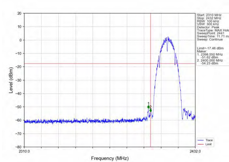
802.11b LCH 2412MHz_Ant1 (SISO)_NTNV
