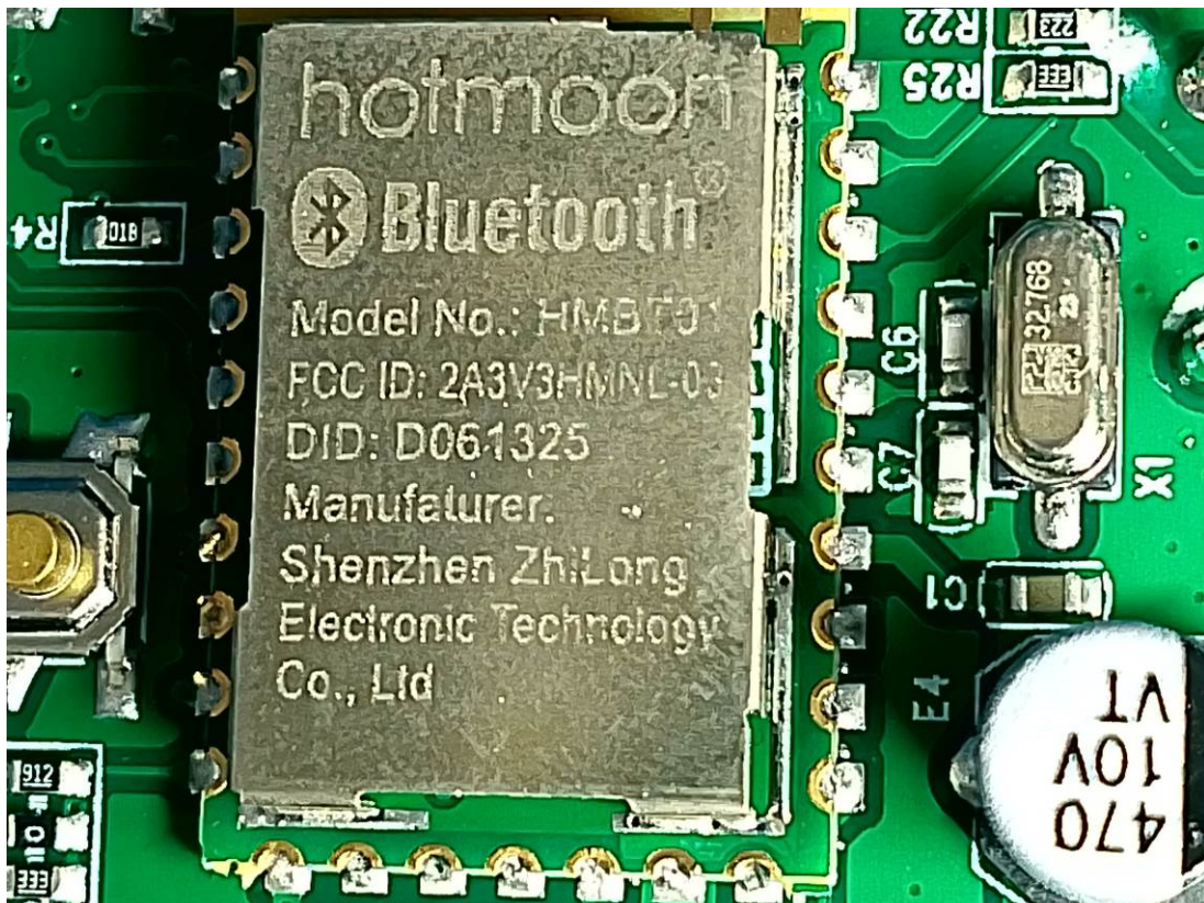
BT Module
