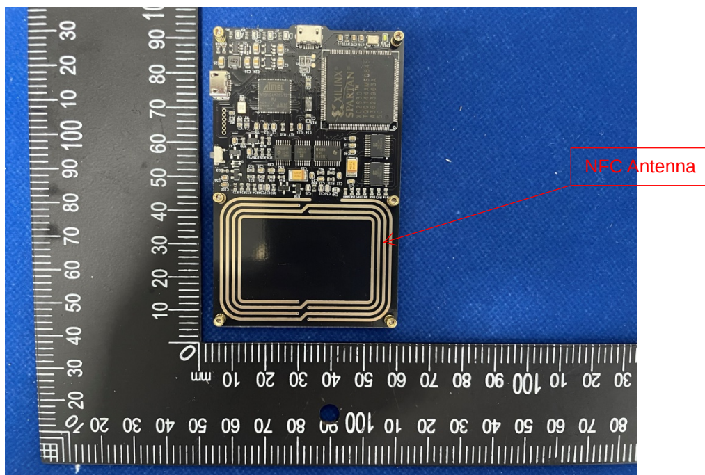
EUT Photo
